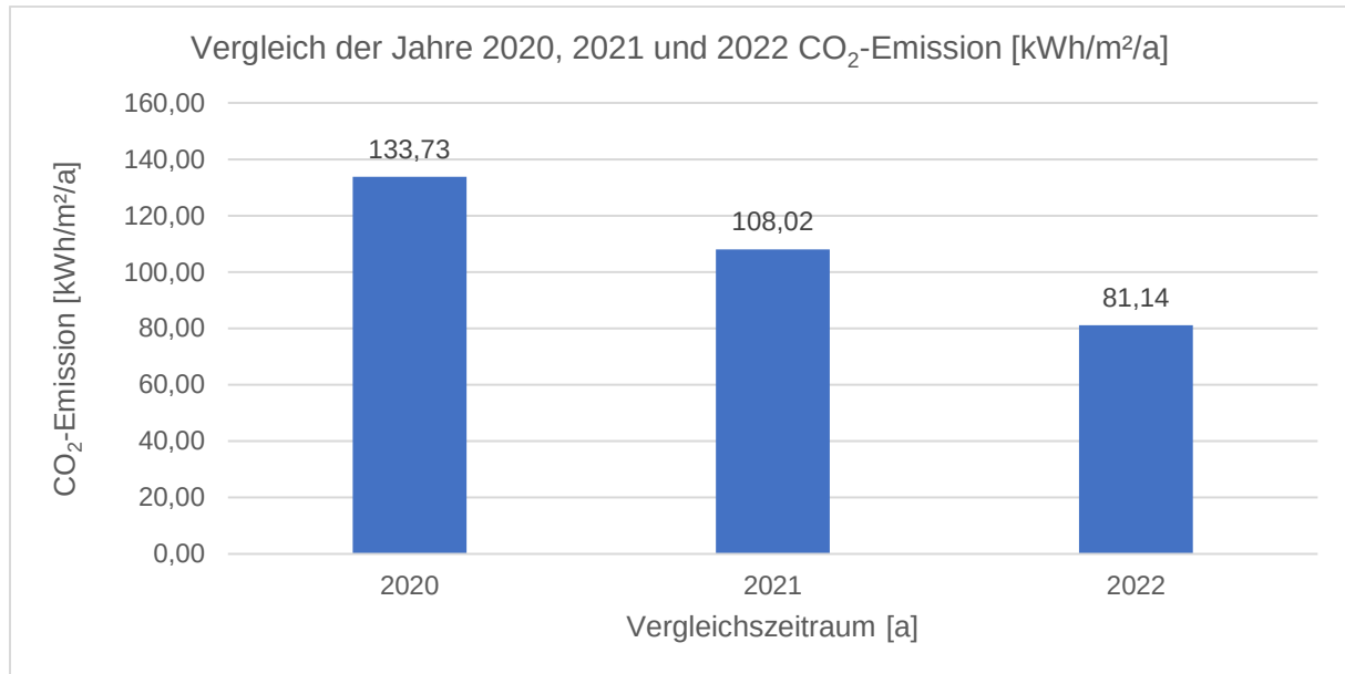
Abbildung 7: Vergleich der Jahre 2020, 2021 und 2022 auf Basis der CO 2 -Emissionen [kWh/m²/a] hinsichtlich der Straßenbeleuchtung (Quelle: eigene Darstellung anhand der Verbrauchsdaten, 2023).
