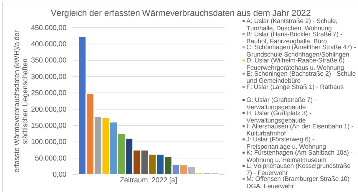
Abbildung 1: Vergleich der Wärmeverbrauchsstärksten Liegenschaften im Stadtgebiet Uslar (Quelle: eigene Darstellung anhand der Verbrauchsdaten, 2023).
