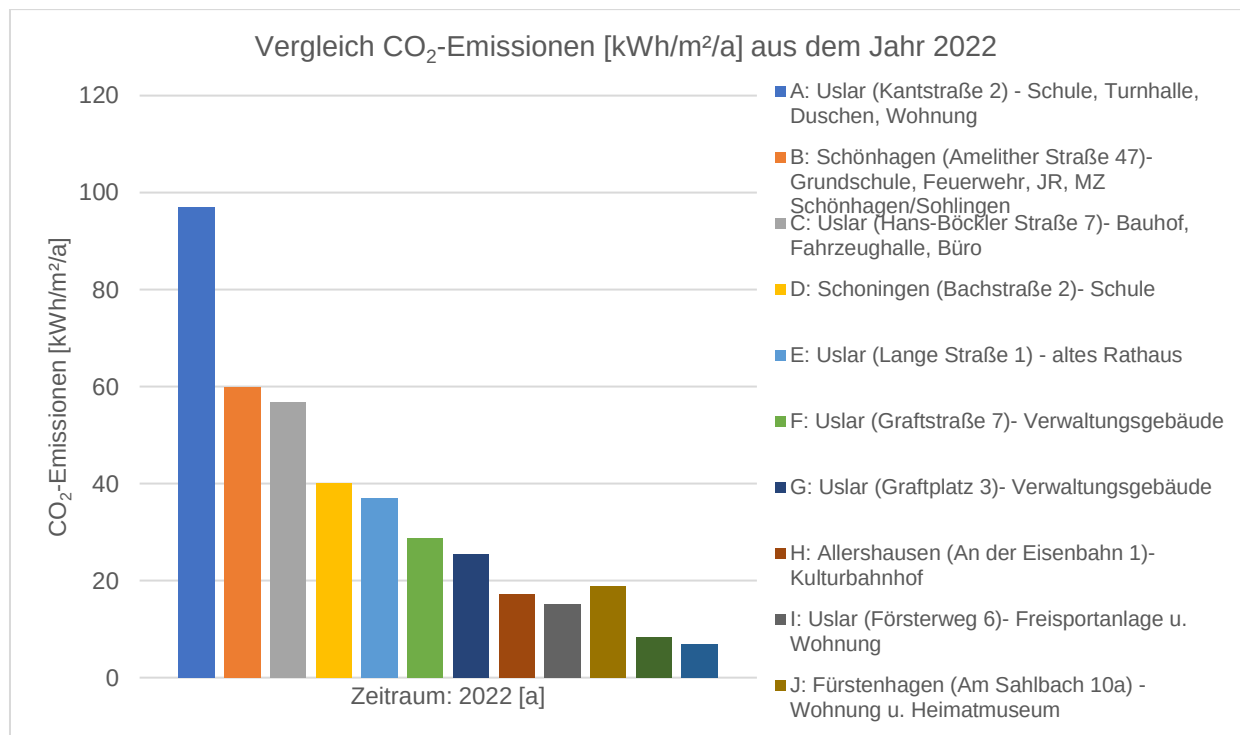
Abbildung 6: Vergleich der verbrauchsstärksten Liegenschaften auf Basis der CO 2 -Emissionen [kWh/m²/a] hinsichtlich der Wärmeverbräuche aus dem Jahr 2022 (Quelle: eigene Darstellung anhand der Verbrauchsdaten, 2023).
